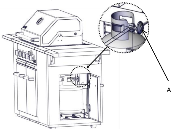
A. Ensemble détendeur/tuyau
