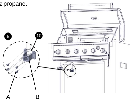
A. 4 vis B. Support de montage à bride 90° en 2 parties
