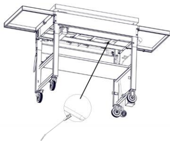
brûleur principal
