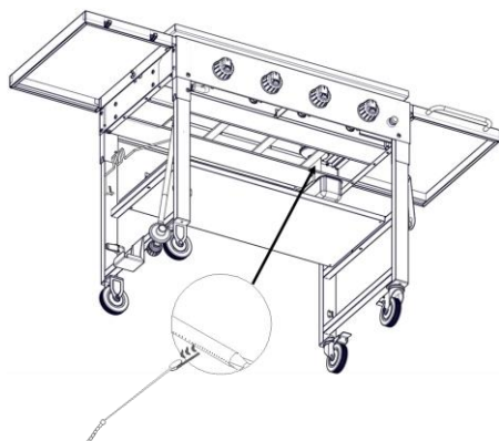
Quemador Principal
