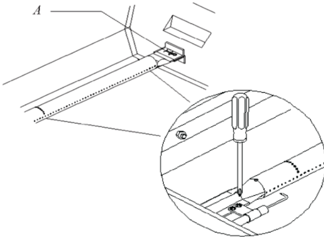
A. Clip
