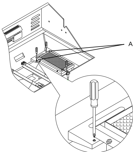
A. 2 Screws
