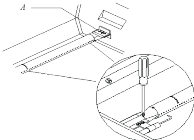
A. Agrafe
