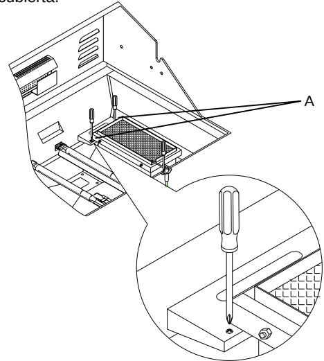
A. 2 tornillos
