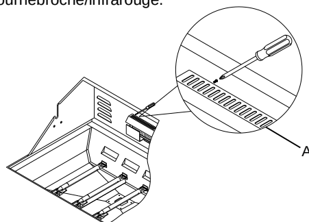
A. Capot coupe-vent
