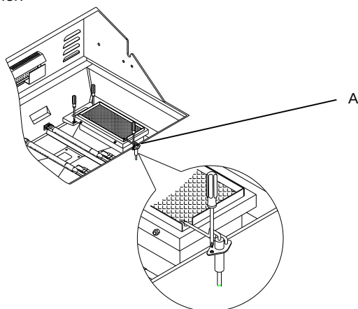
A. Screw
