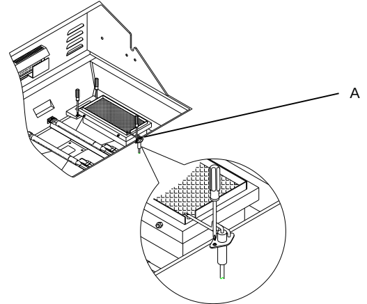
A. Tornillo
