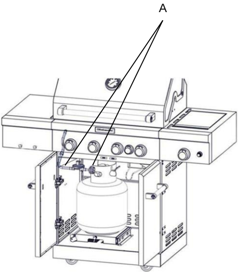
A. Ensemble détendeur/tuyau
