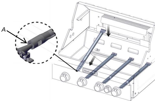
A. Conexión del quemador/orificio
