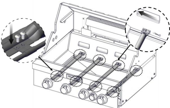
A. Conexión del quemador/orificio
