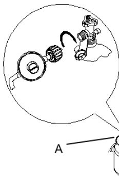
A. Ensamblaje de regulador de presión/manguera de gas B. Tanque de gas combustible LP de 20 lb
