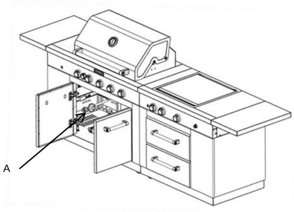
A. Ensemble détendeur/tuyau
