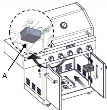
A. Plateau d'égouttement
