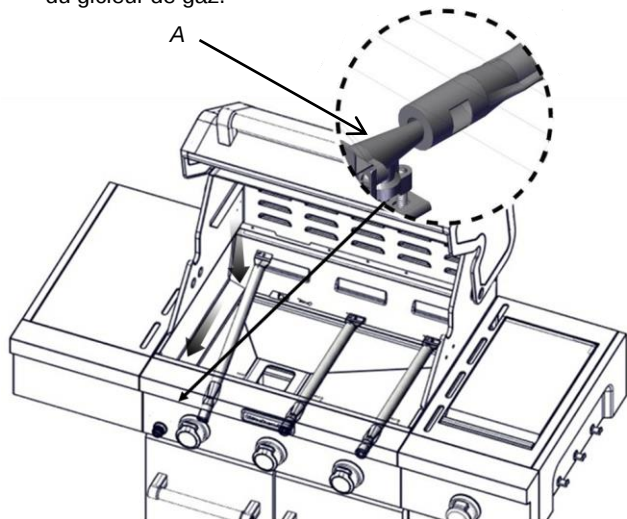
A. Burner / connexion orifice
