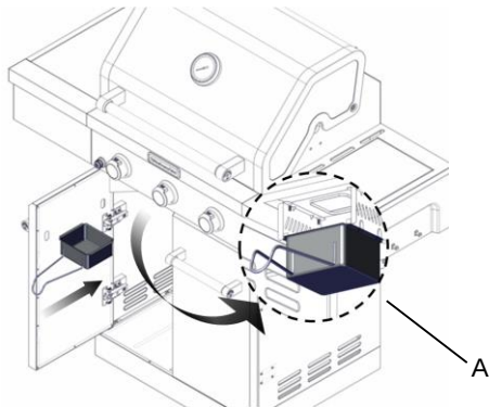
A. Grease Box
