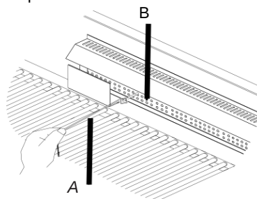
A. Extensión de encendido B. Quemador trasero para sellar
