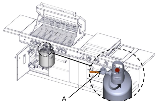
A. Assemblage du régulateur de pression de gaz/du tuyau
