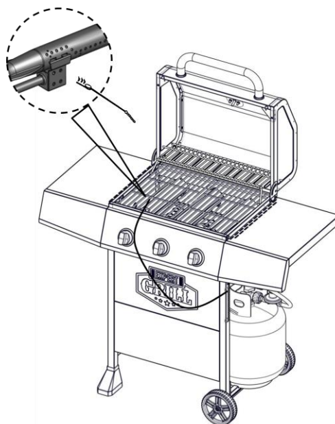
Brûleur principal
